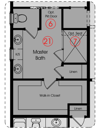
Optional Master Bath
